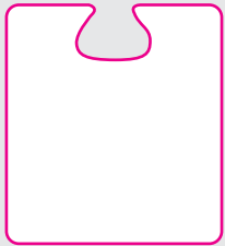
Nose Die (Watt) 95mm x 105mm
